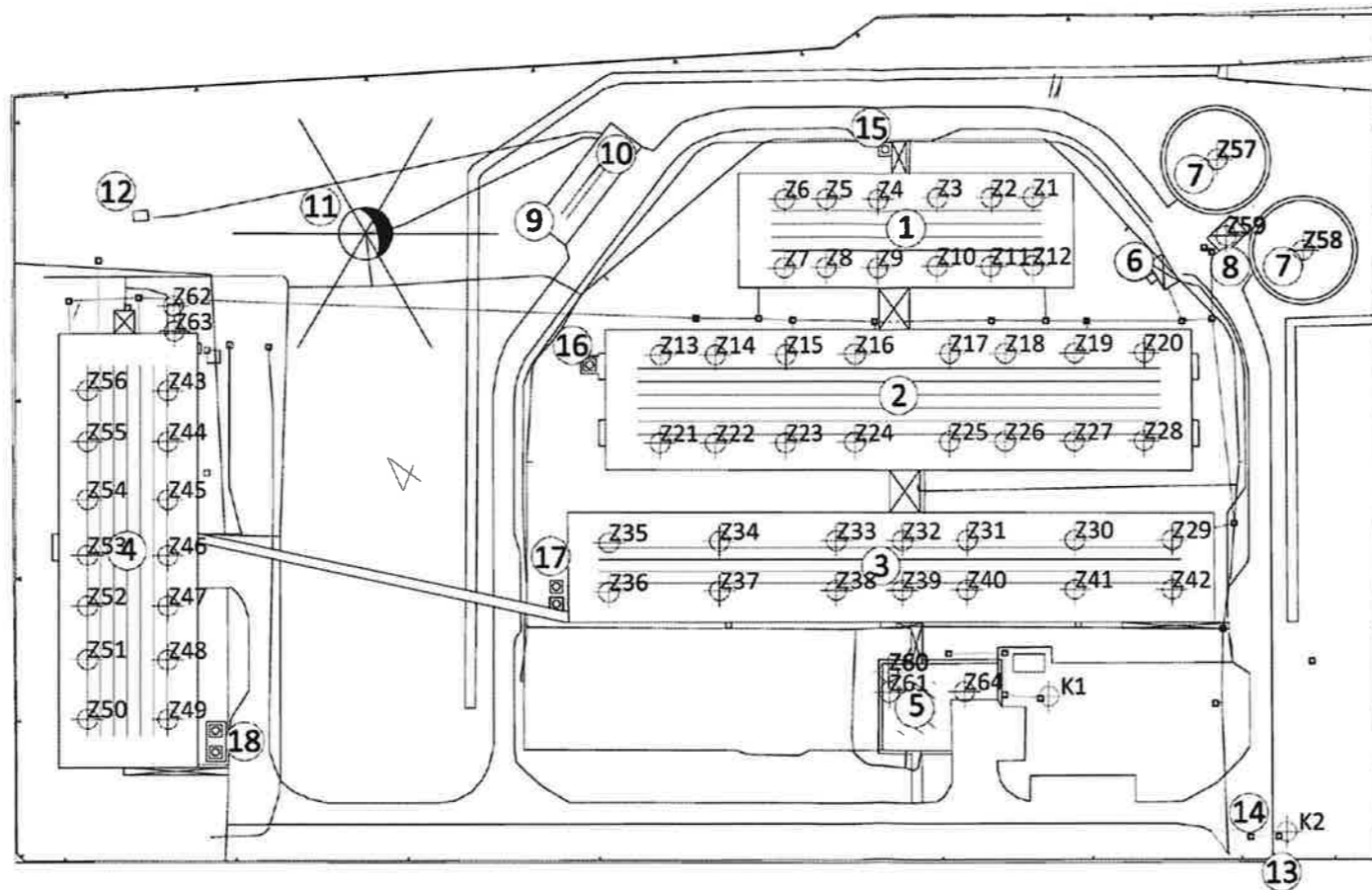
Prilog 1. Situacija sa prikazom objekata, mjesta emisija i sustava vodoopskrbe i odvodnje na lokaciji farme Malo Kneževo.
